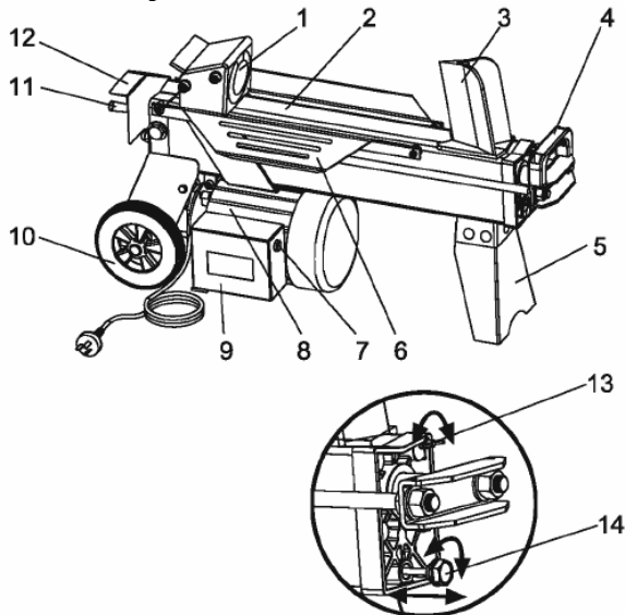
Abb. 1: PREHLS52 / 042001 PREHLS52/5 / 042031
