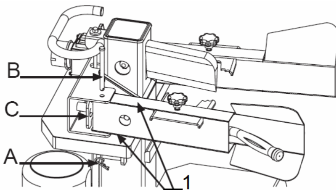
Fig.6 : (1) Applicare lubrificante
