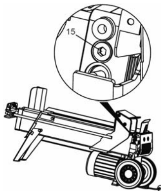
Fig.12 : PREHLS7T / 042011
