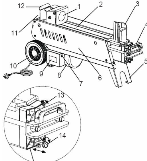
Abb. 2 : PREHLS7T / 042011
